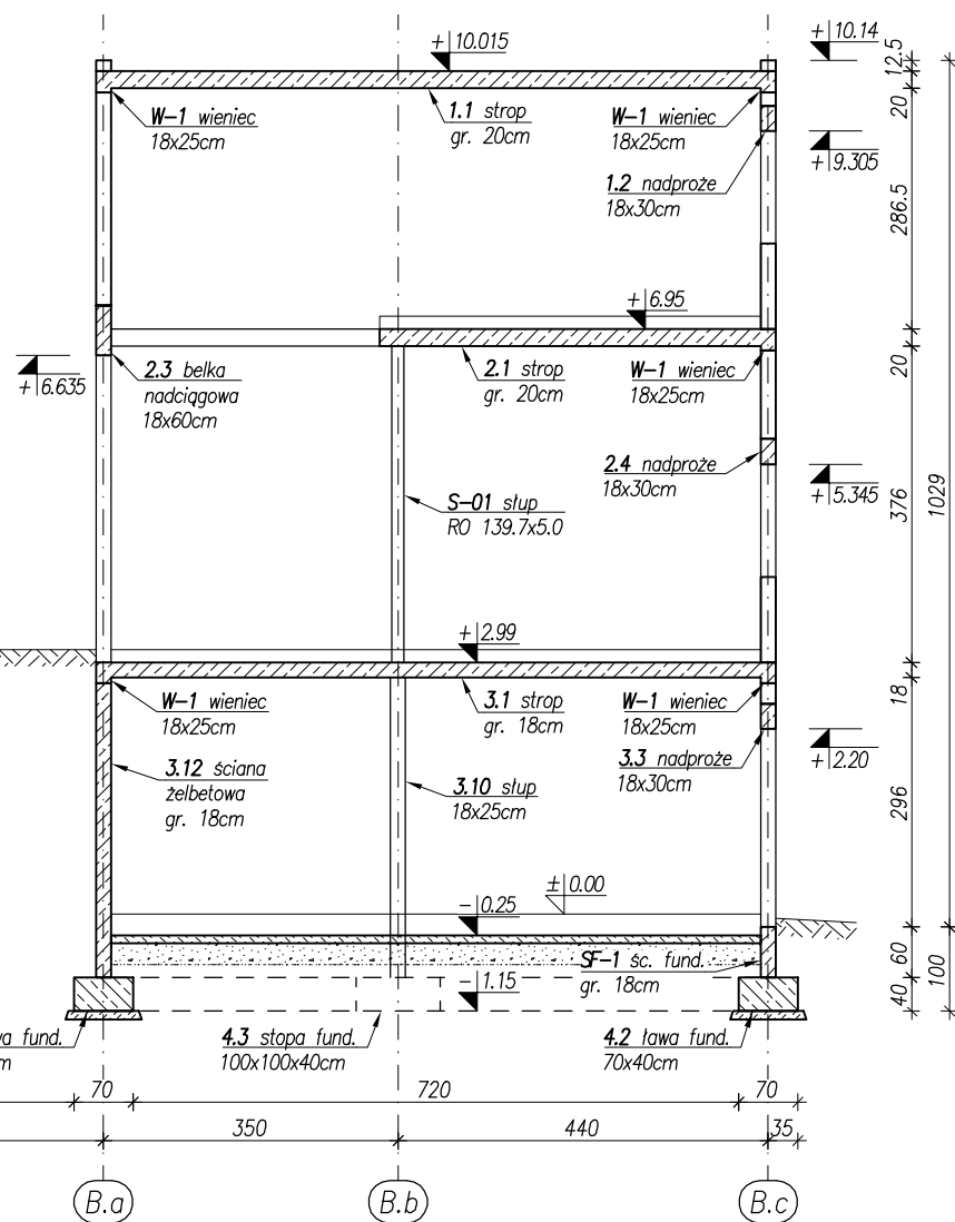
przekrój B-B
