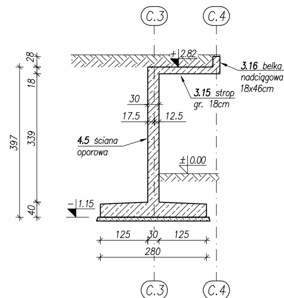
przekrój 1-1
