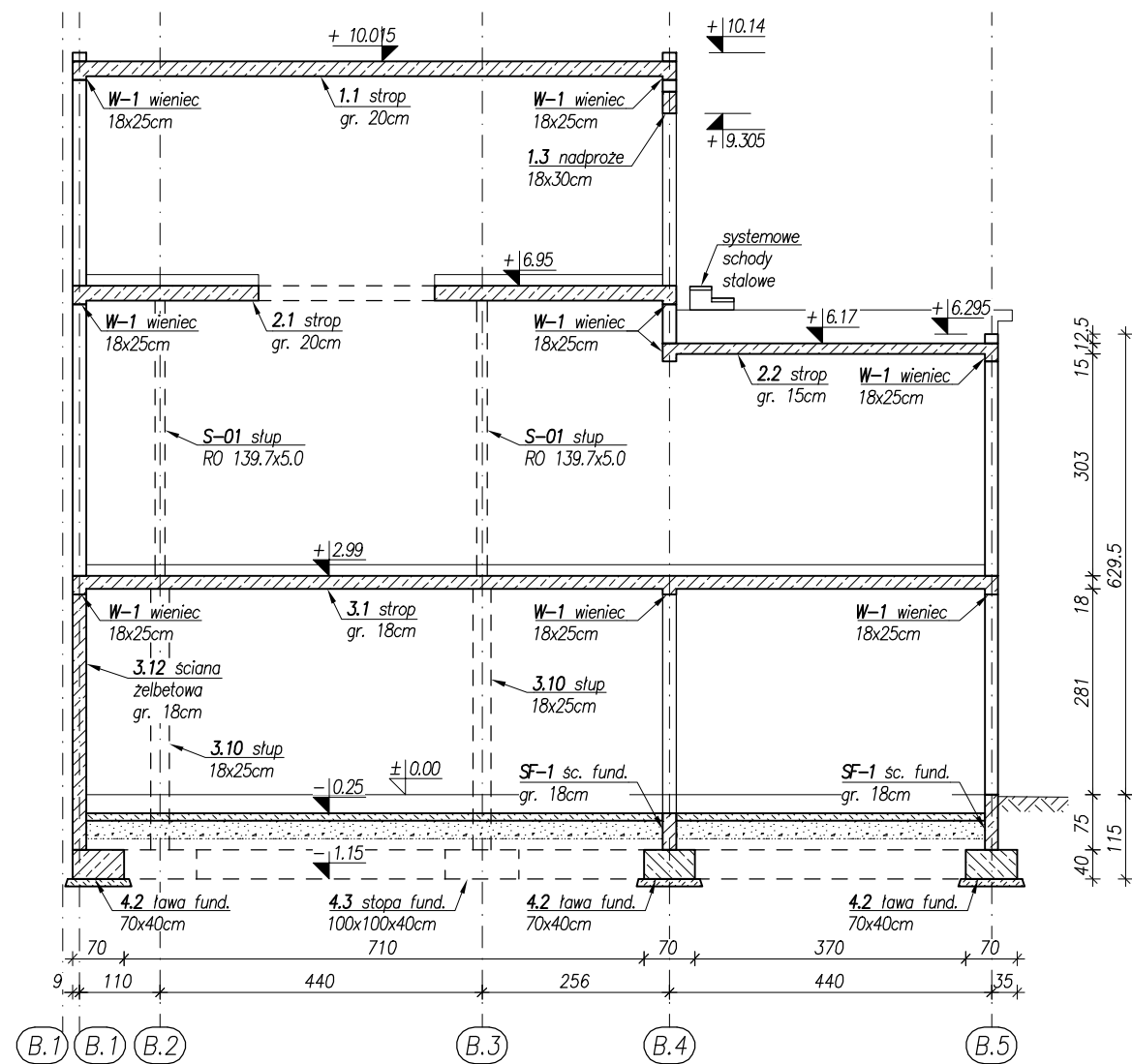
przekrój A-A
